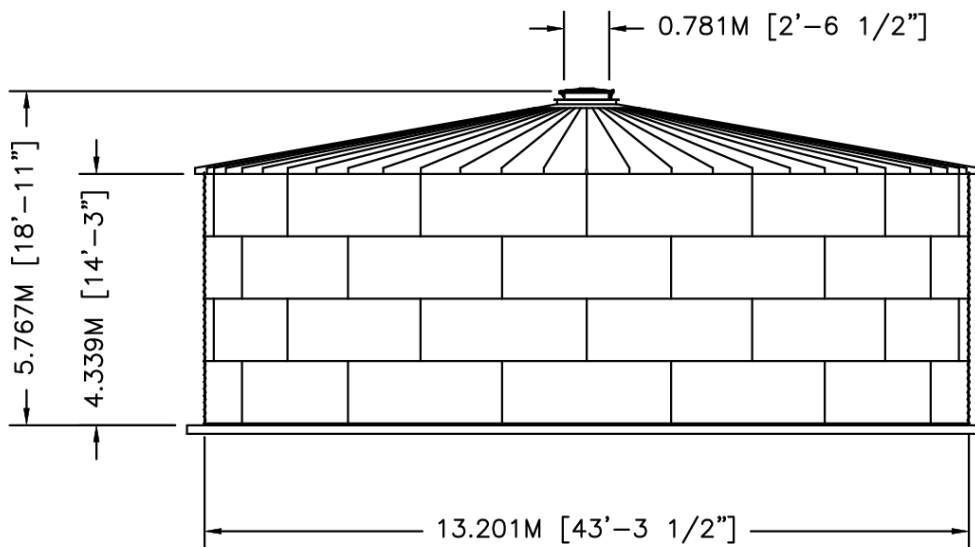
ELEVATION
